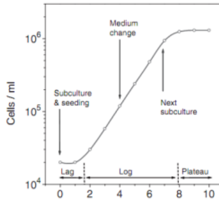
Gambar 5. Kurva Pertumbuhan
